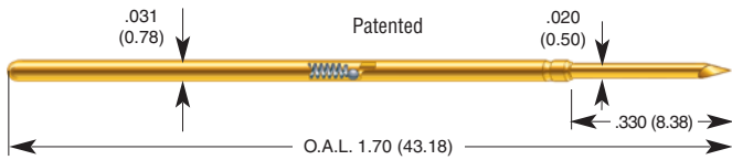
POGO-72J POGO-72J-S
