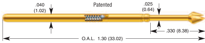
POGO-1J POGO-1J-S
